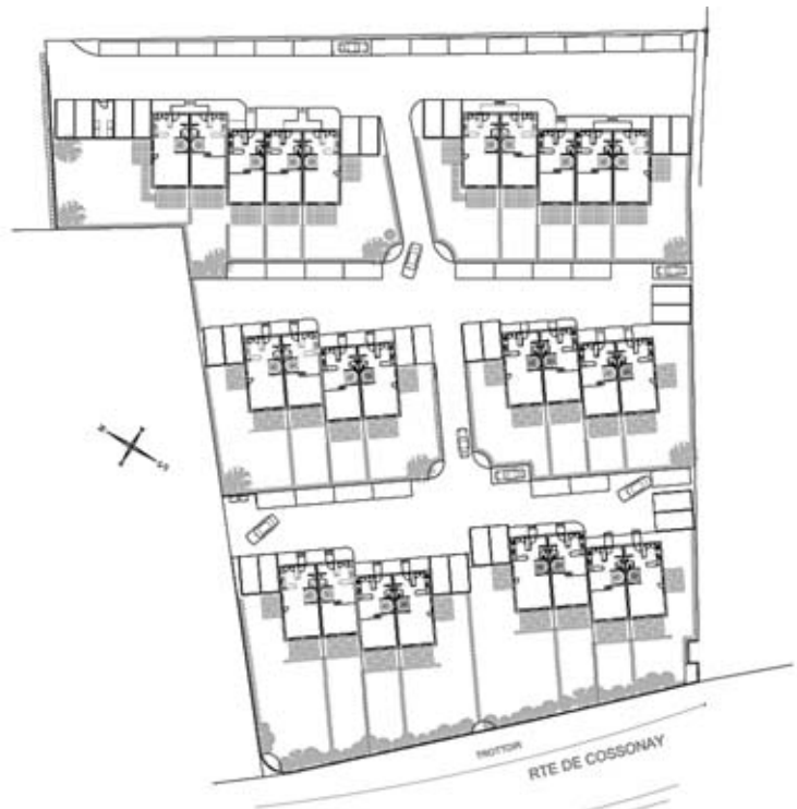
Plan masse
