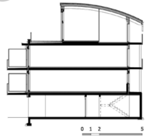
Coupe transversale
