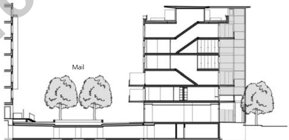
Coupe transversale
