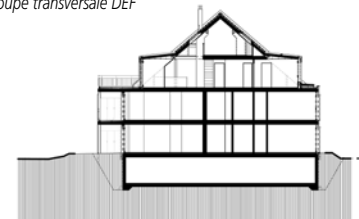
Coupe transversale DEF
