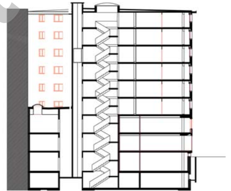
Coupe transversale
